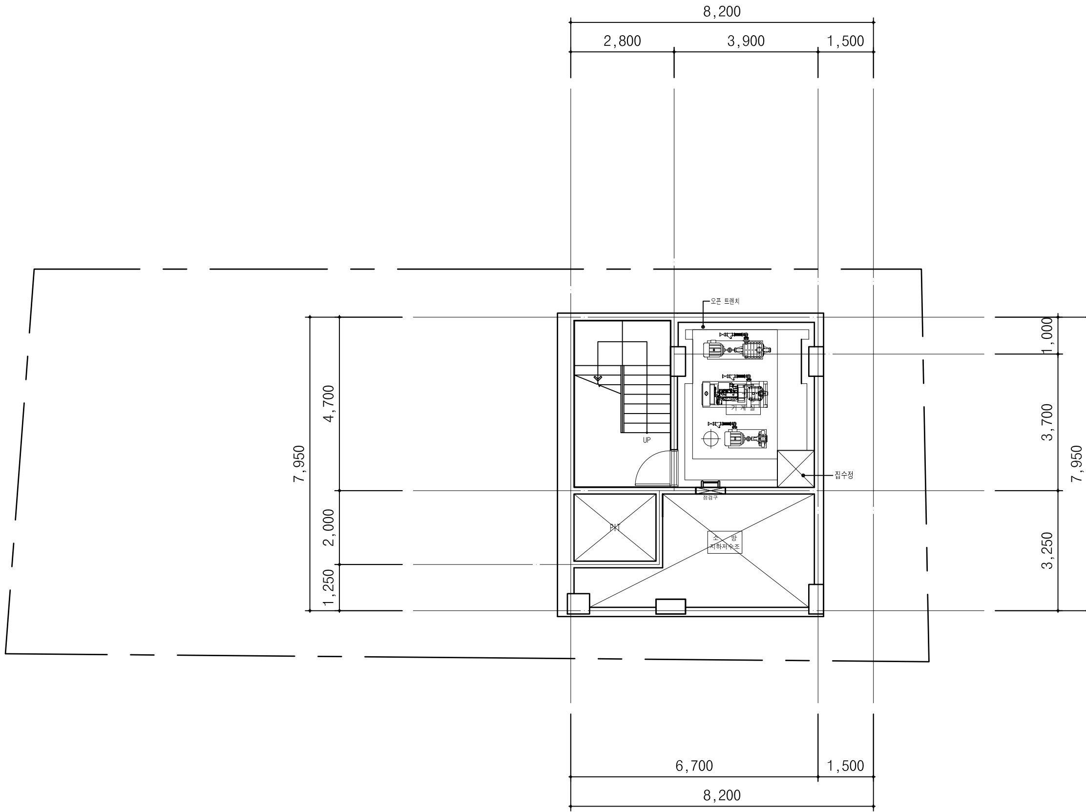
지하1층 평면도 SCALE : A3 : 1/100
