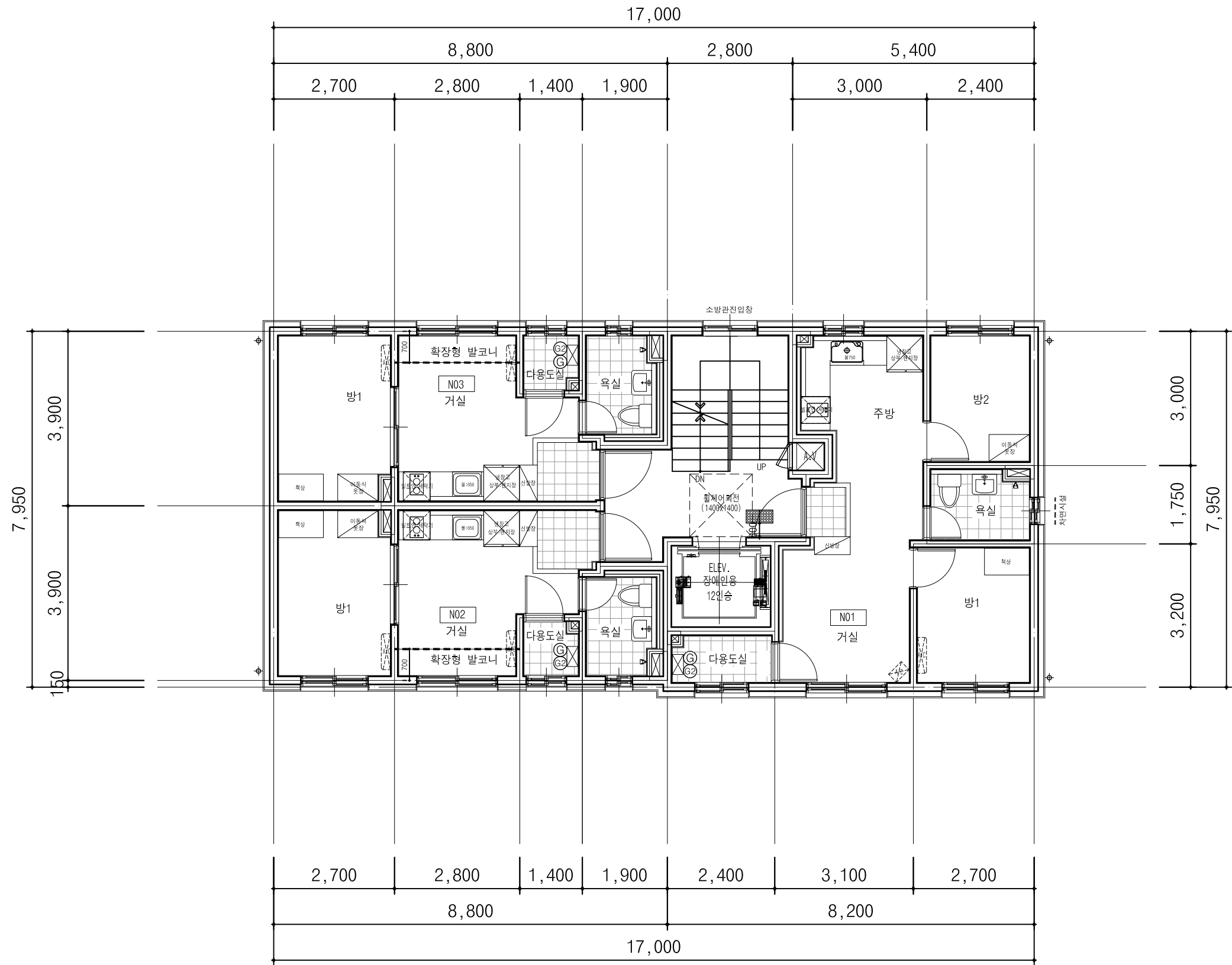
2 층 평면도 SCALE : A3 : 1/100
