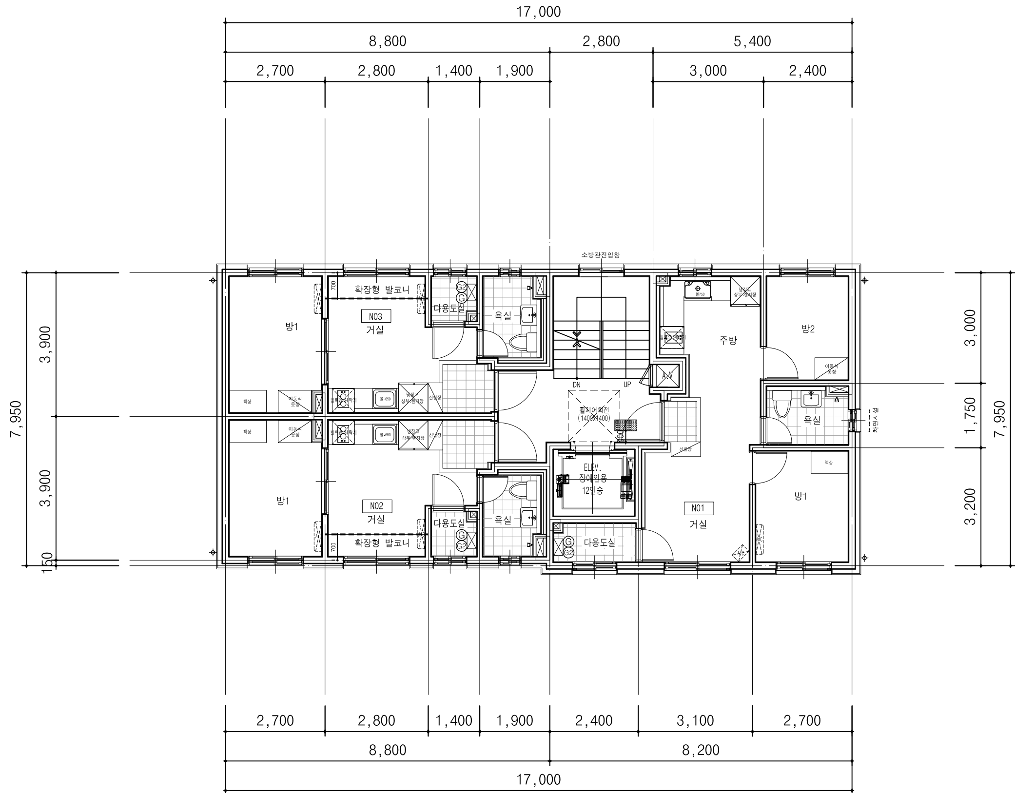
3~6 층 평면도 SCALE : A3 : 1/100
